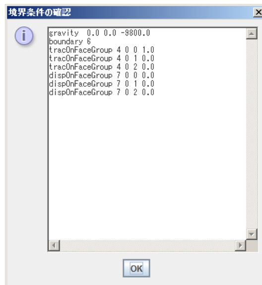
図 6.3-15 境界条件の確認
