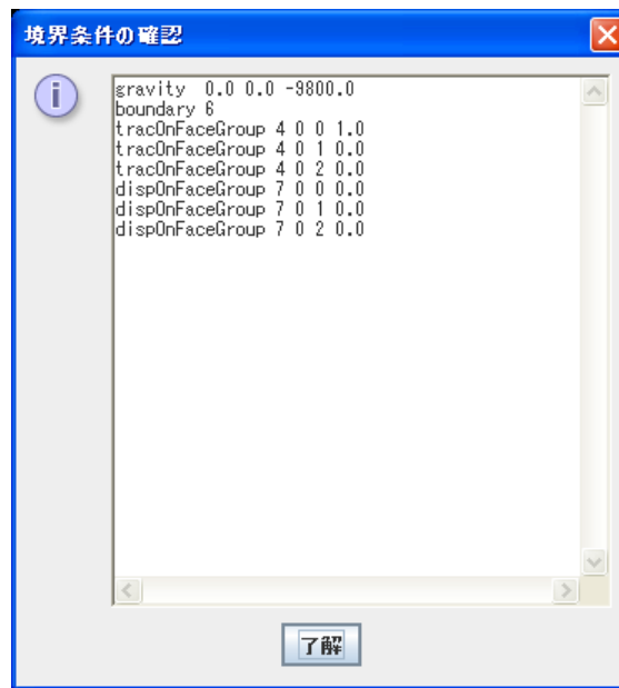
図 7.3-2 境界条件の確認
