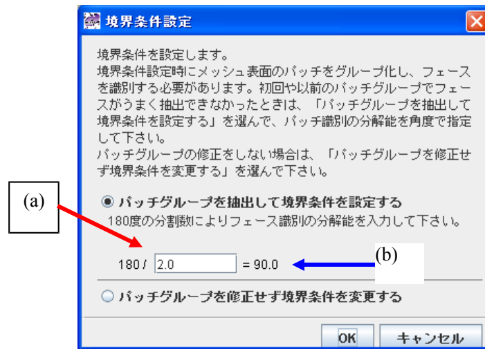
図 6.3-4 メッシュのフェースのグループ化パラメータの入力
